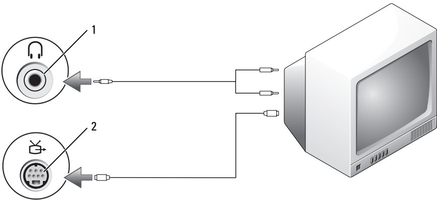
1 Audioanschluss 2 S-Video-TV-Ausgang
