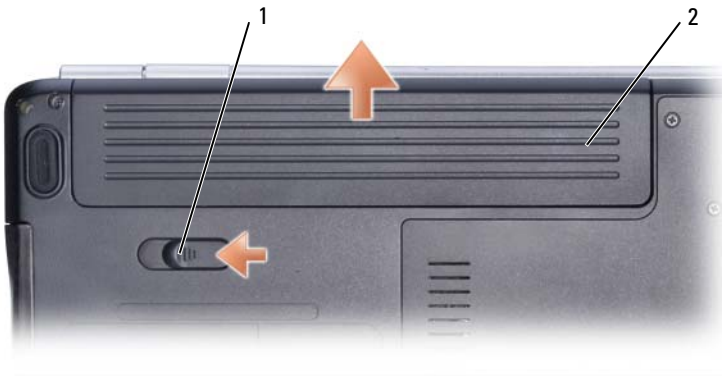
1 Riegel der Akkufach- Freigabevorrichtung 2 Akku
