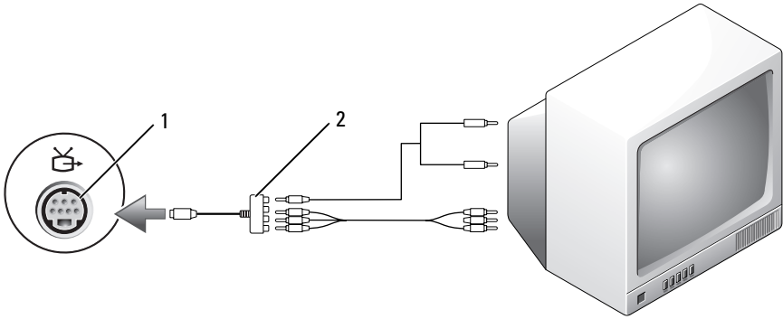
1 S-Video-TV-Ausgang 2 Komponenten-Video-Adapter
