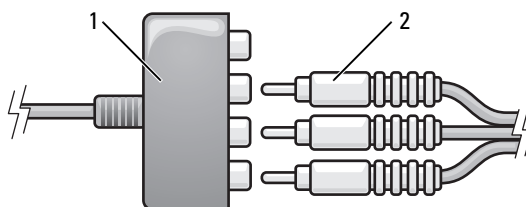
1 Komponenten-Video-Adapter 2 Komponenten-Video-Kabel
