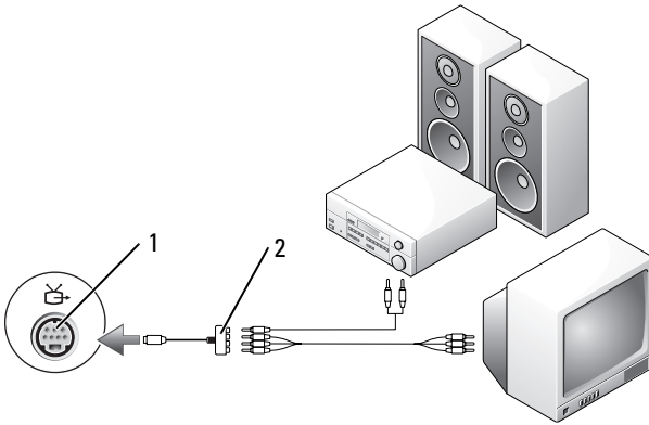
1 S-Video-TV-Ausgang 2 Komponenten-Video-Adapter
