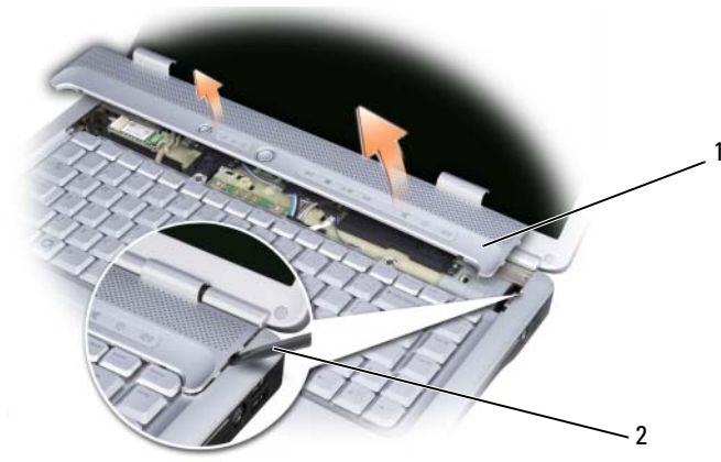
1 Scharnierabdeckung 2 Stift
