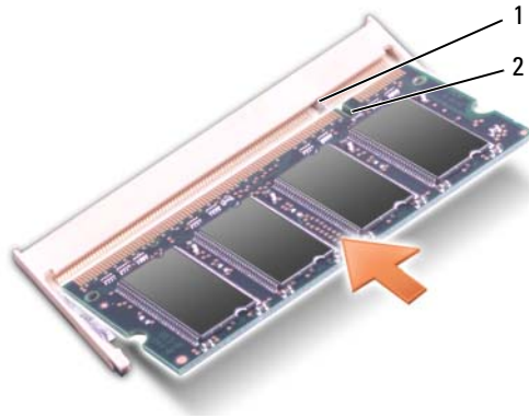
1 Zapfen 2 Kerbe
