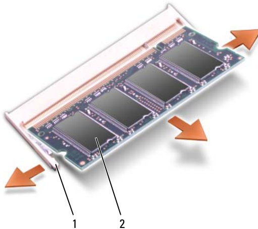
1 Sicherungsklammern (2) 2 Speichermodul
